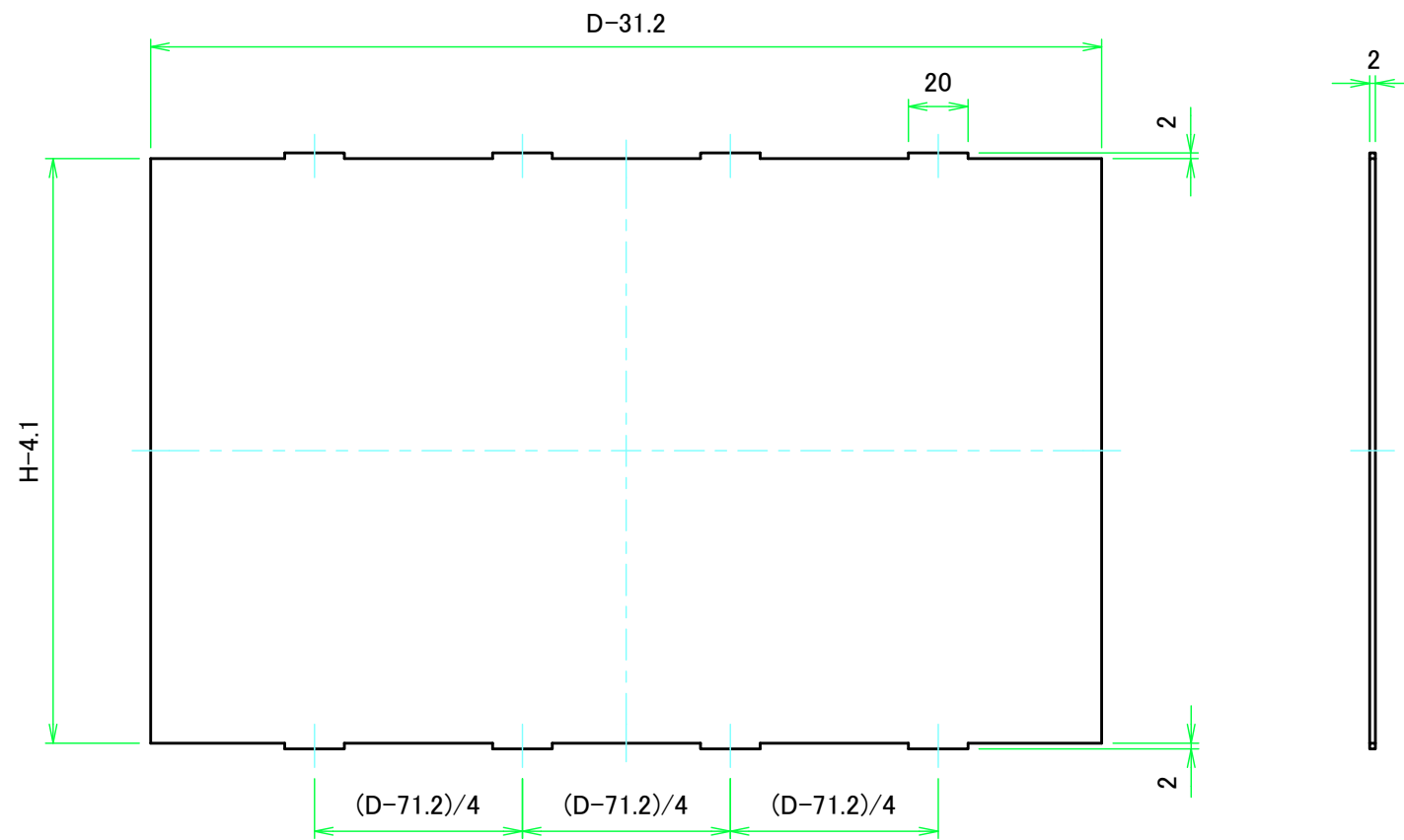
Dパネル1表面 / D Panel 1 Frontside
