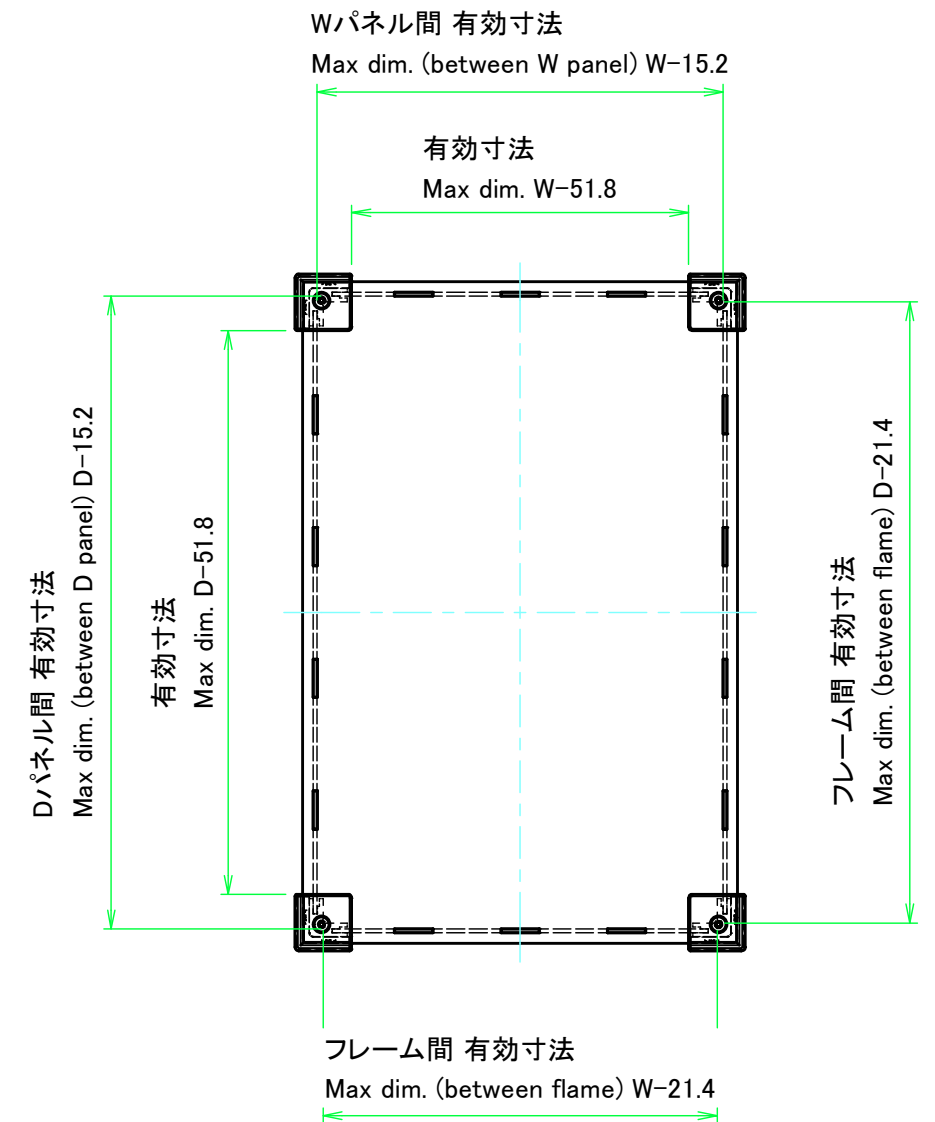
下カバー / Bottom cover
